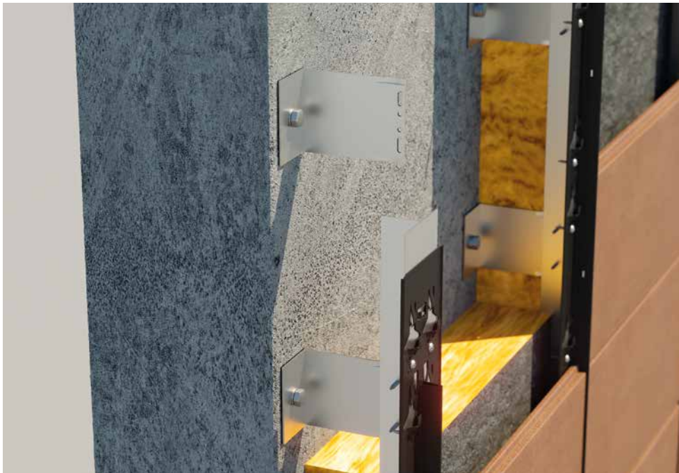
Systemprofil / T-Profil
